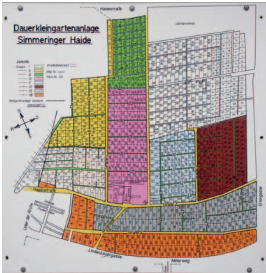
Slika 100: Načrt velikega območja vrtnikov Simmeringer Haide na Dunaju.
