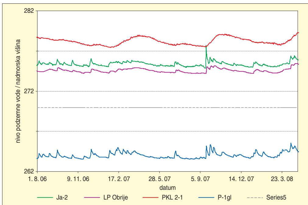
Slika 52: Raven podzemne vode na območju vodarne Jarški prod (LP Ja-2), Kleče (PKL 2-1) in Hrastje (LP Obrje) ter na območju Zaloga (P-1gl) med avgustom 2006 in aprilom 2008.
