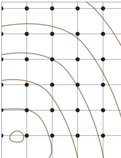
Slika 1: Točkovni digitalni model reliefa s pravilno mrežo kvadratov.
