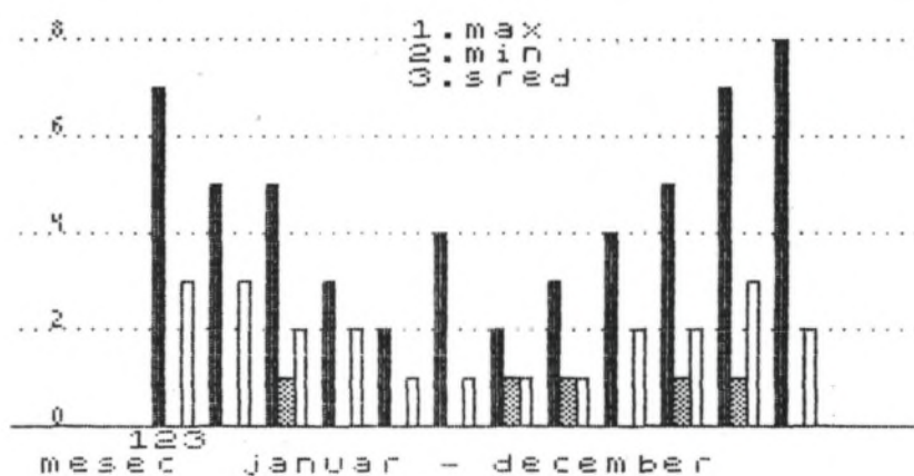
RAVNE - ČEČOVLJE 1984 koncentracija dima mg/m 3 x 100
