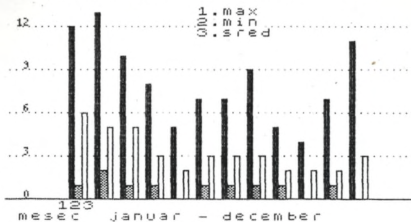
RAVNE-ČEČOVLJE 1984 koncentracija SO 2 mg/m 3 x 100
