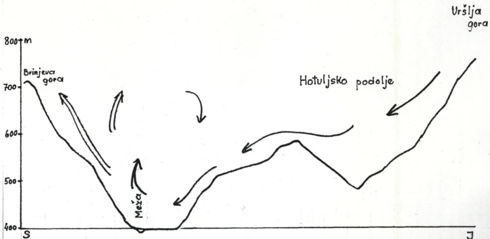
Risba 3 Lokalna značna cirkulacija v Sp. Mežiški dolini
