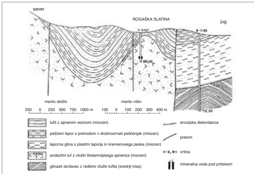
Slika 2: Prečni geološki prerez Rogaške Slatine (Nosan 1973, 34).
